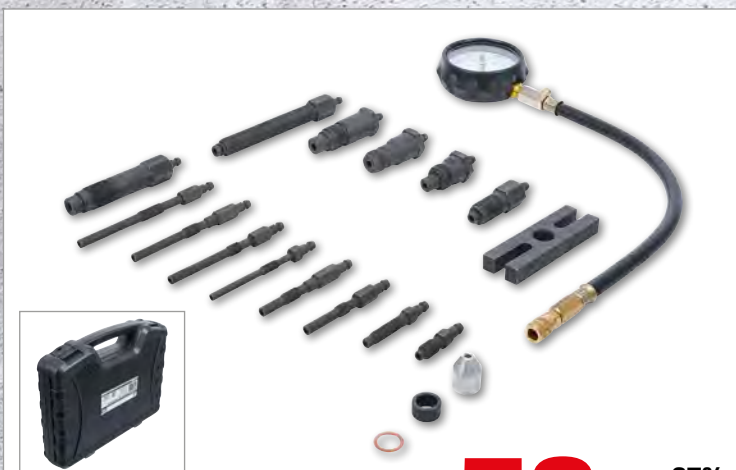
Kompressionstester für Dieselmotoren
