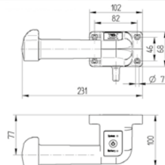
EDUZ300: Rechte Handbedieneinheit mit Funktion.
