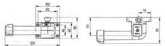
EDFZ300: Rechte Handbedieneinheit mit Funktion und Not-Halt-Schalter.
